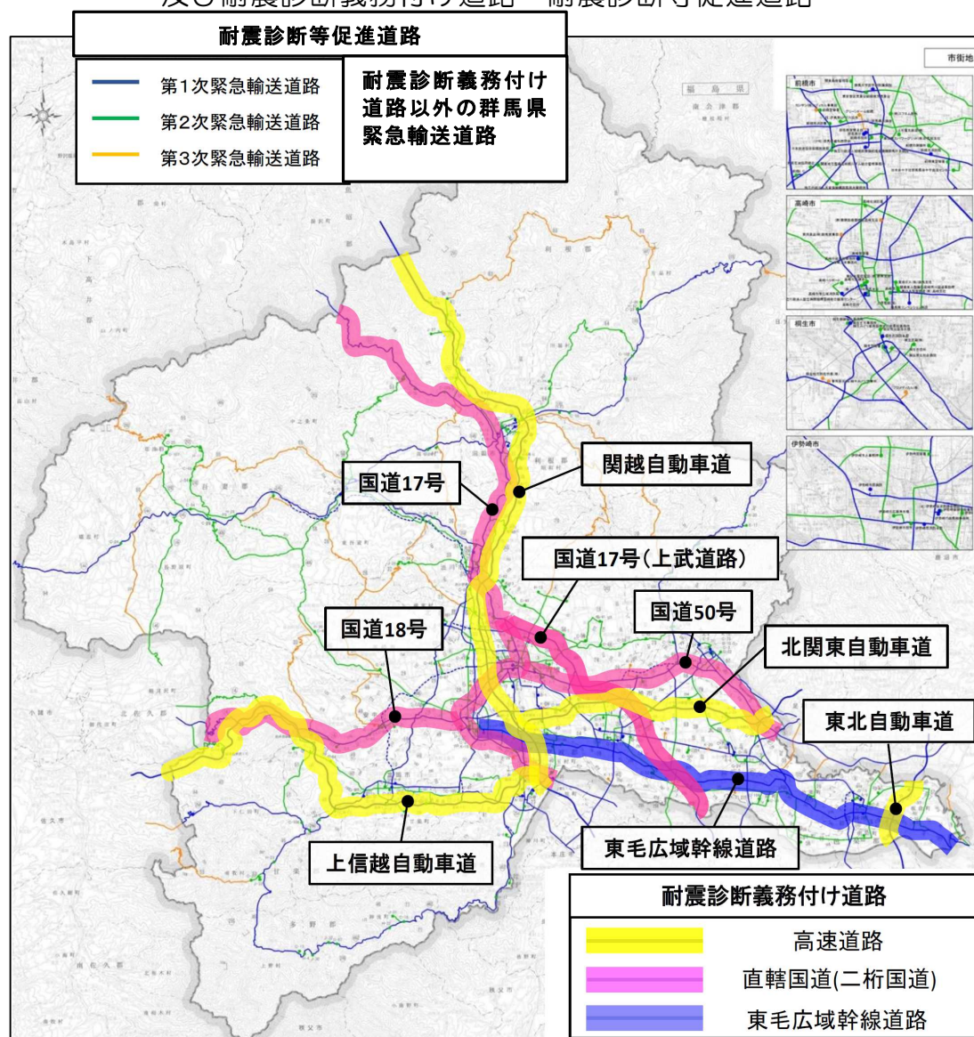
(図4-5) 群馬県緊急輸送道路ネットワーク図 及び耐震診断義務付け道路・耐震診断等促進道路
