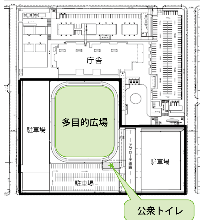
多目的広場・公衆トイレ等工事配置図
